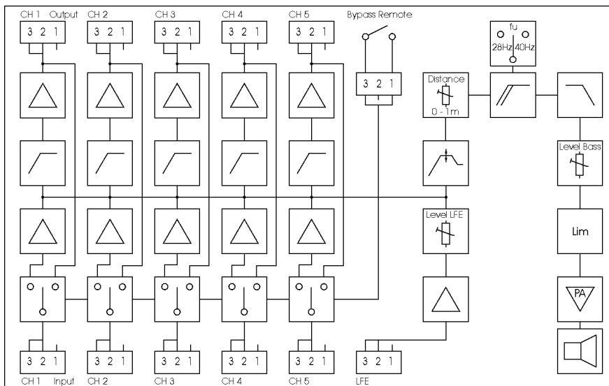
Blockschaltbild
